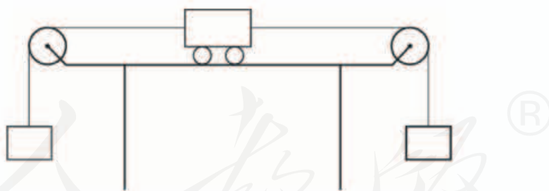
图8.2-2 研究二力平衡条件的一种方法
