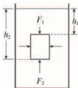
图10.1-3 水对长方体上、下表面的压力不同
