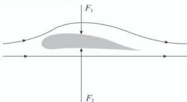
图9.4-4 飞机升力产生的示意图
