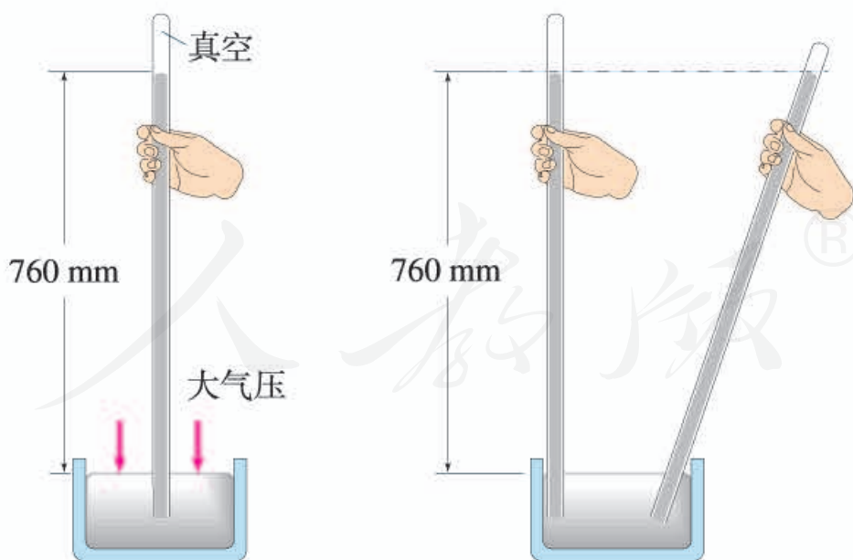
图9.3-3 托里拆利实验
