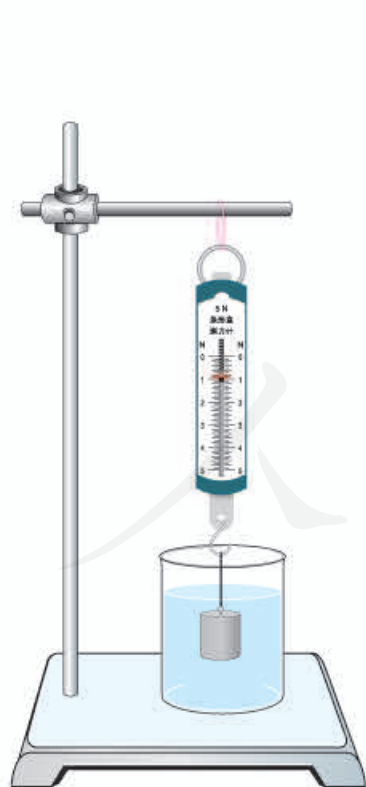
图10.1-5 浮力的大小是否跟物体浸没的深度有关？
