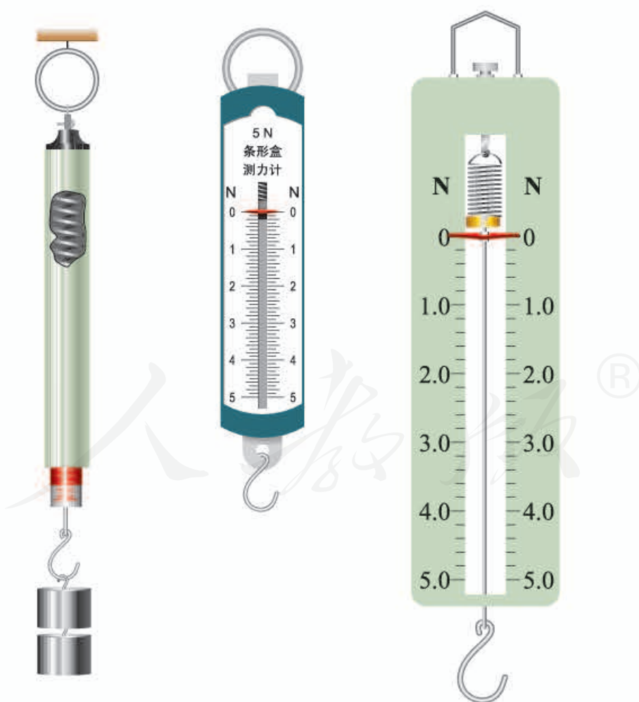
图7.2-2 弹簧测力计
