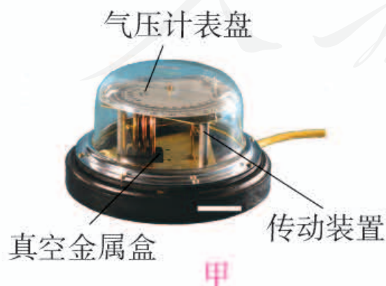
图9.3-4 无液气压计
