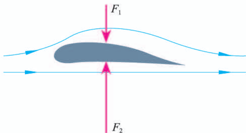
图9.4-4 飞机升力产生的示意图
