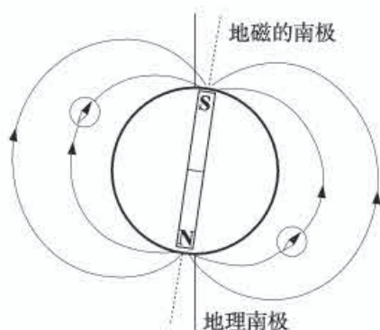
图 20.1-9 地球是一个巨大的磁体
