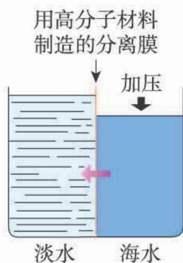
图12-12 用高分子分离膜淡化海水
