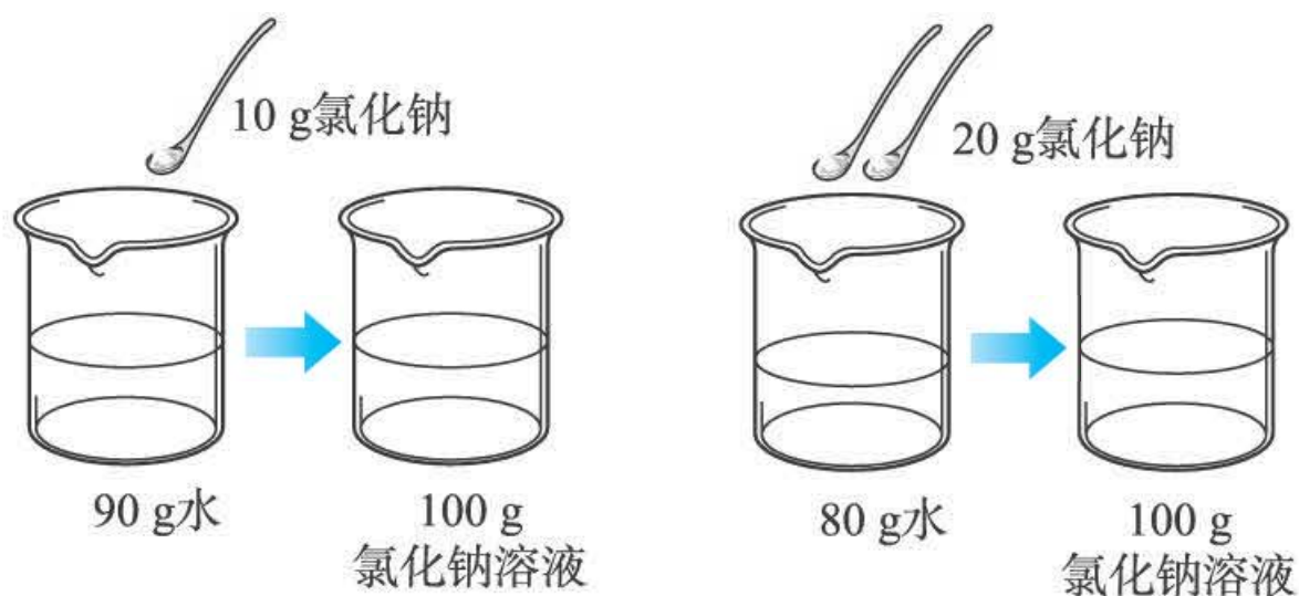
图9-10 配制两种质量分数不同的氯化钠溶液
