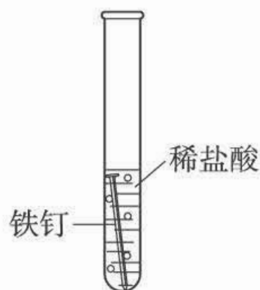
图8-3 金属在稀盐酸中
