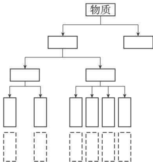
图11-3 物质的分类
