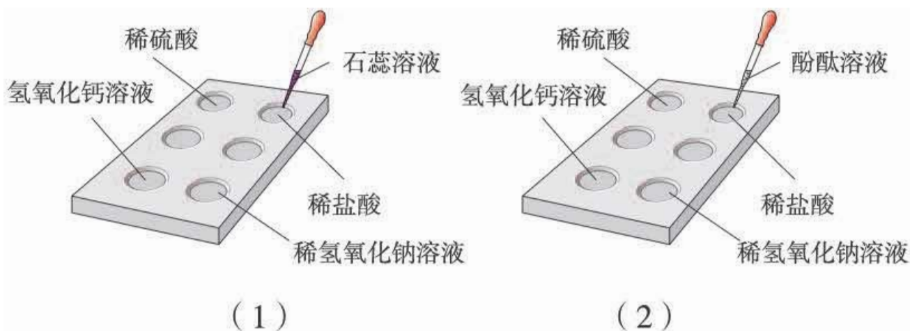
图10-15 酸、碱与指示剂作用
