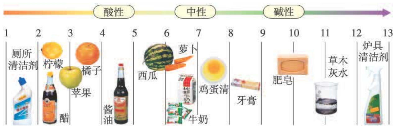
图10-14 身边一些物质的pH
