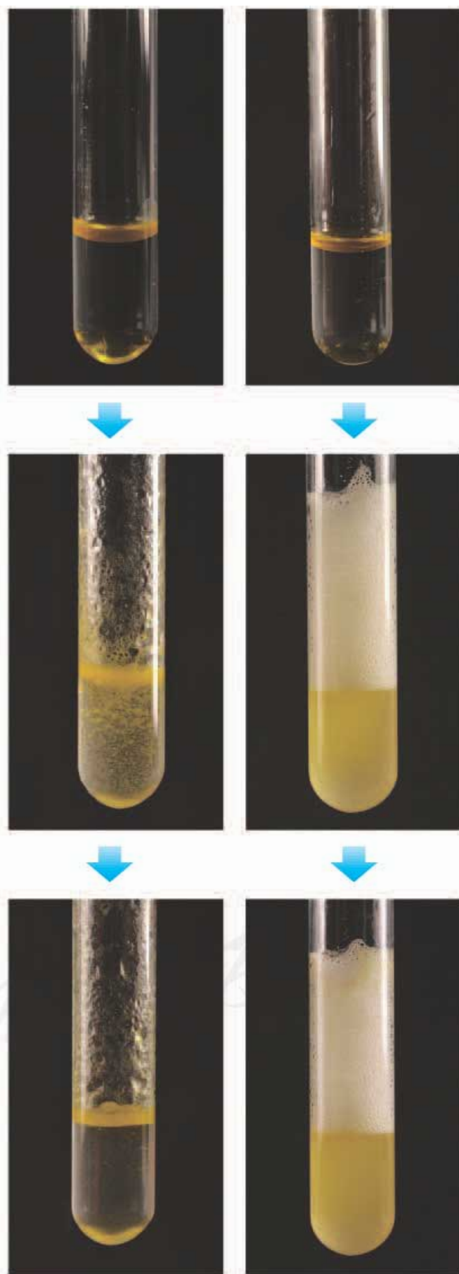
图9-4 乳浊液的形成和乳化现象
