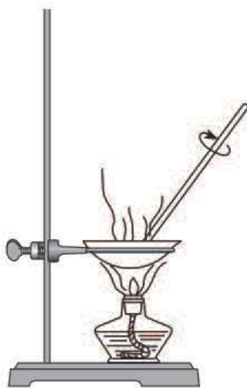
图11-6 蒸发食盐水
