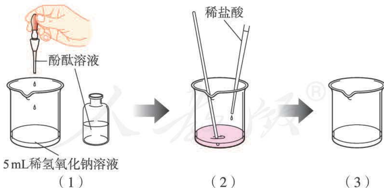
图10-9 在氢氧化钠溶液中滴加稀盐酸
