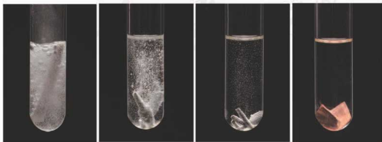
图8-4 镁与稀盐酸的反应
