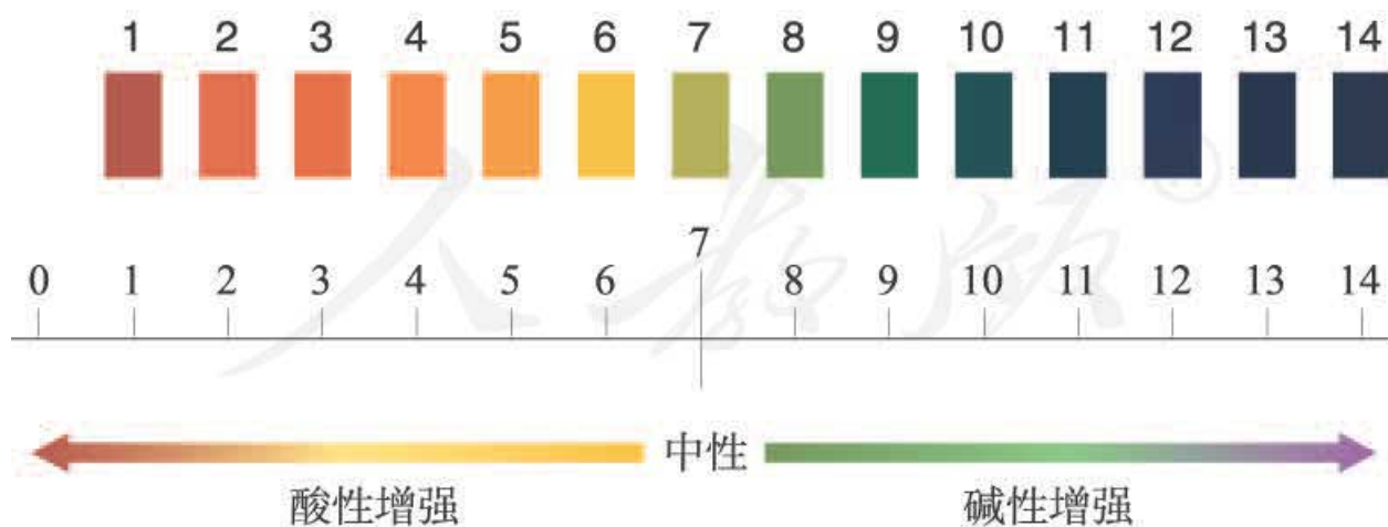
图10-12 pH和溶液的酸碱性
