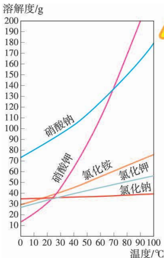
图9-7 几种固体物质的溶解度曲线 图9-8 氢氧化钙的溶解度曲线
