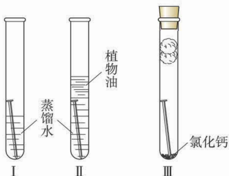
图8-15 铁钉锈蚀条件的探究
