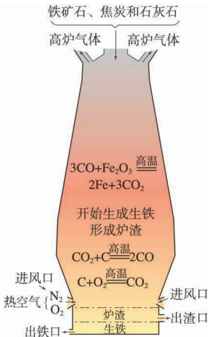
图8-14 炼铁高炉及炉内化学反应过程示意图
