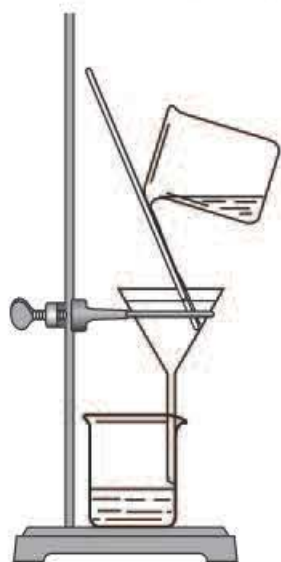
图11-5 过滤食盐水
