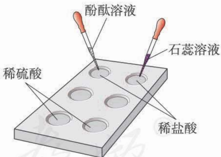
图10-5 酸与指示剂作用
