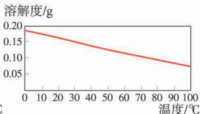
图9-7 几种固体物质的溶解度曲线 图9-8 氢氧化钙的溶解度曲线
