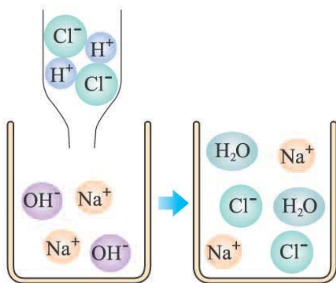
图10-10 氢氧化钠与盐酸反应示意图
