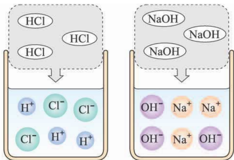
图10-7 HCl和NaOH在水中解离出离子
