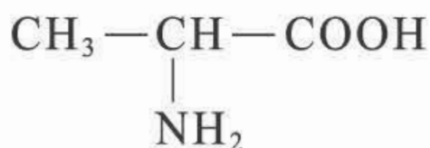
图12-1 丙氨酸
