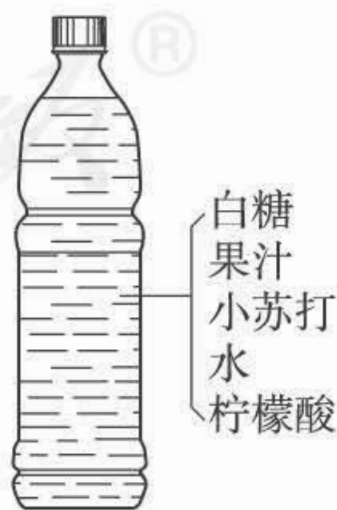
图9-11 自制汽水
