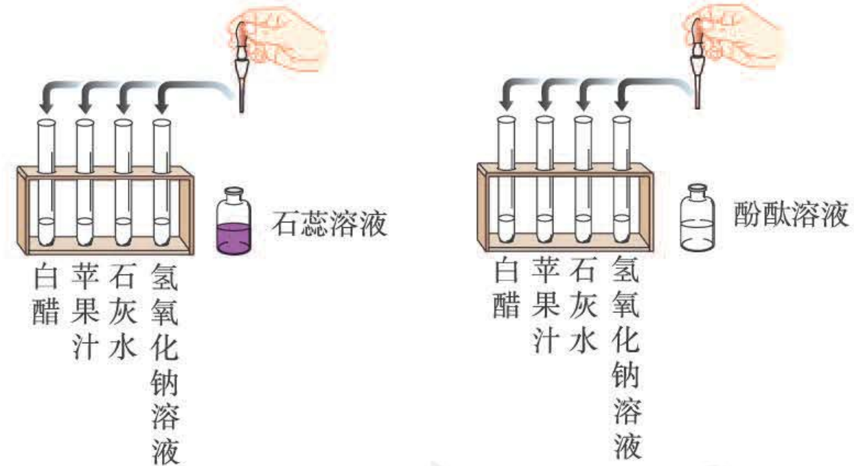
图10-1 向溶液中加入酸碱指示剂
