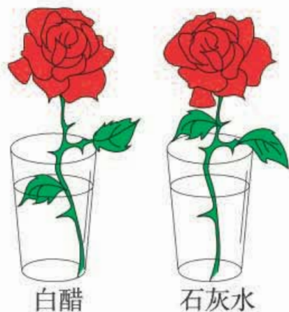
图10-8 酸或碱溶液能改变花的颜色
