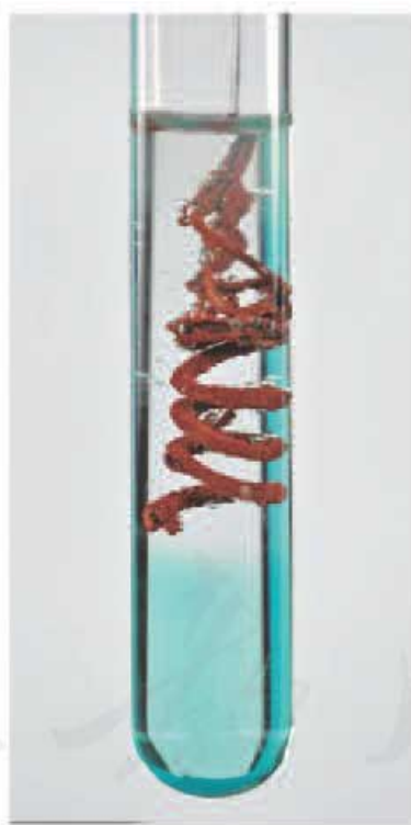
图8-8 铝与硫酸铜溶液的反应
