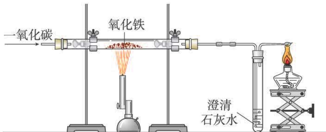
图8-13 一氧化碳还原氧化铁
