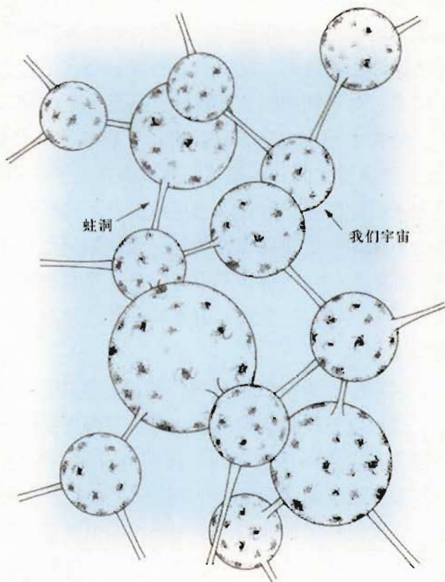
我们宇宙或许是无数个平行宇宙中的一个。每一个宇宙通过无穷多的虫洞（连通两个时空域的隧道）跟其他宇宙相连。在这些虫洞之间旅行是可能的，但可能性又微乎其微。
