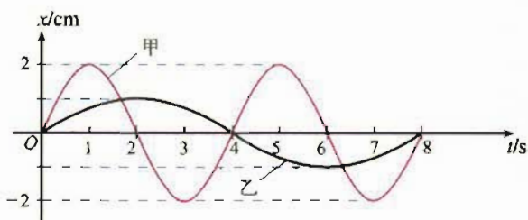
图 11.4-8 两个单摆的振动图象
