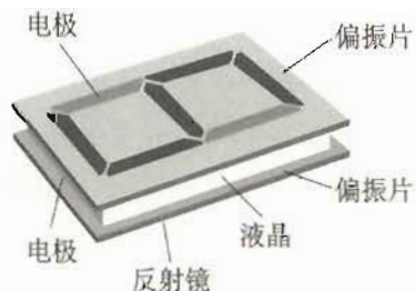
图 13.6-6 液晶显示用到了偏振光
