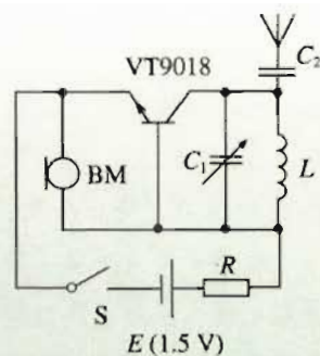
图 14.3-5 无线话筒电路图
