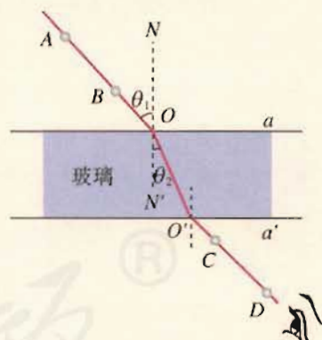
图13.1-3 测定玻璃的折射率
