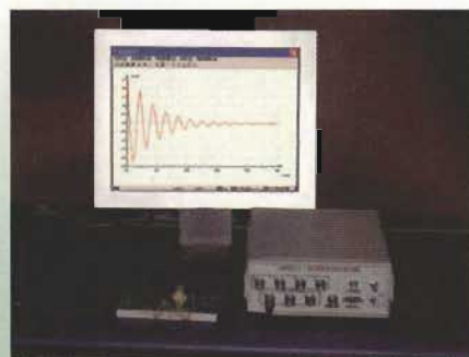
图 14.2-3 用传感器观察振荡电流
