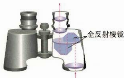
图 13.2-5 双筒望远镜中的全反射棱镜
