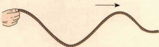
图 12.1-2 沿绳传播的波
