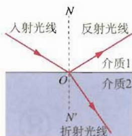
图 13.1-1 光的反射和折射同时存在
