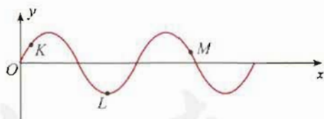
图12.2-4 某简谐横波的图象
