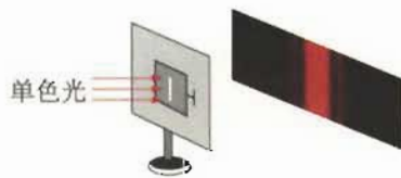
图 13.5-1 单缝衍射示意图
