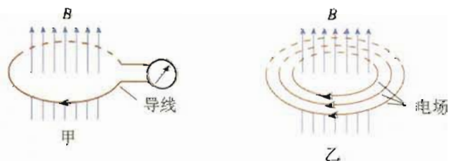
图 14.1-1 变化的磁场产生电场
