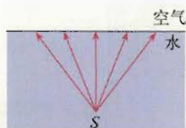
图 13.2-11 水下的点光源
