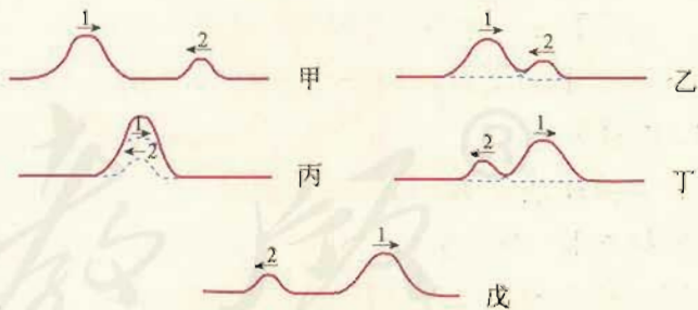
图 12.4-3 波的叠加
