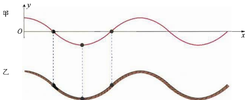
甲 横波的图象 乙 绳上的横波
