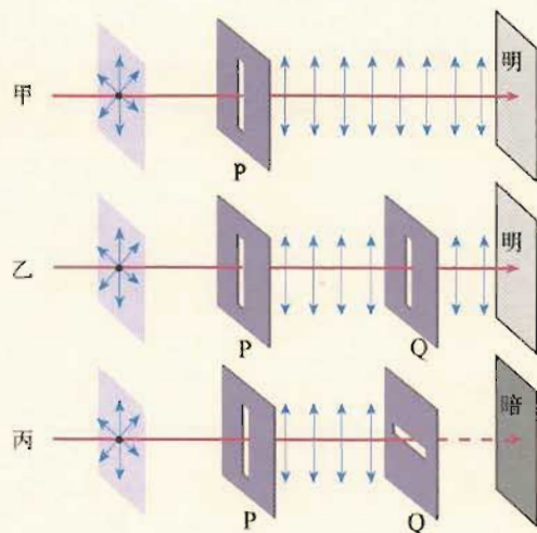
图 13.6-2 检验光波是不是横波
