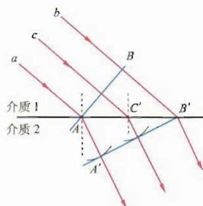
图 12.6-6 用惠更斯原理研究波的折射
