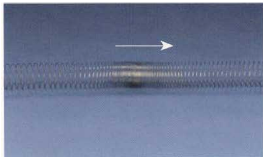
图 12.1-5 纵波的形成
