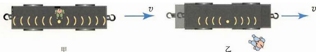
图 15.2-1 闪光是否同时到达前后两壁?
