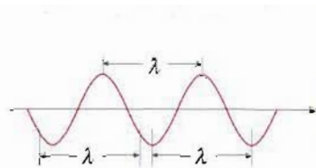
图 12.3-1 波长
