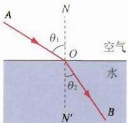
图 13.1-2 光的折射
