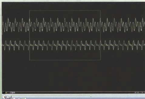
图 11.2-4 比较两个声音的频率
