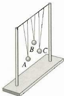
图 11.5-8 判断摆的运动
