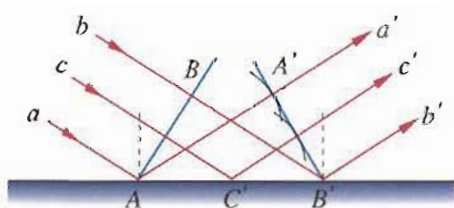
图 12.6-5 用惠更斯原理解释波的反射
