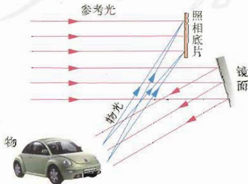
图 13.8-2 全息照片的拍摄
