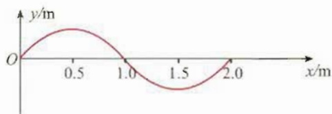
图12.2-5 沿 x 轴正方向传播的横波
