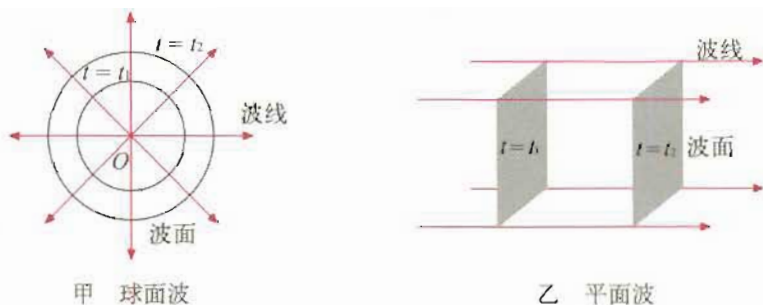
图12.6-1 波面与波线
