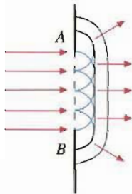
图 12.6-4 用惠更斯原理解释波的衍射
