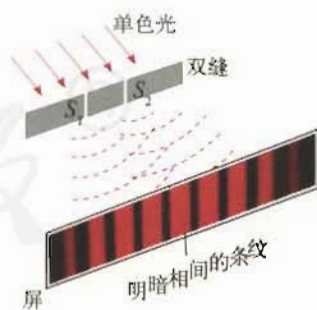
图 13.3-2 杨氏双缝干涉的示意图
