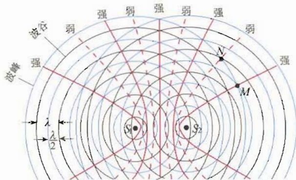
图 12.4-5 波的干涉的示意图
