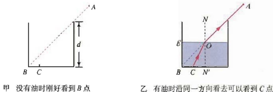
图 13.1-4 计算油的折射率和油中的光速
