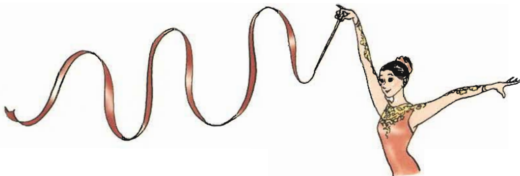
图 12.1-1 彩带飞舞，是振动在彩带上的传播。
