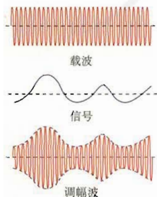
图 14.3-2 调幅
