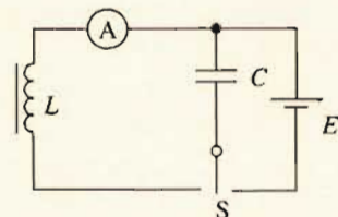
图 14.2-1 产生电磁振荡的电路
