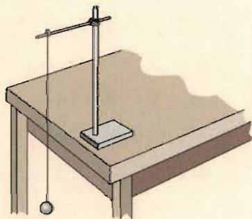
图 11.4-5 测量不同摆长的单摆的周期
