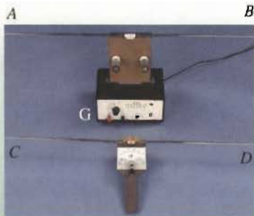
图 14.1-5 演示电磁波发射与接收的装置
