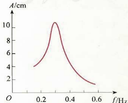
图 11.5-9 单摆的共振曲线
