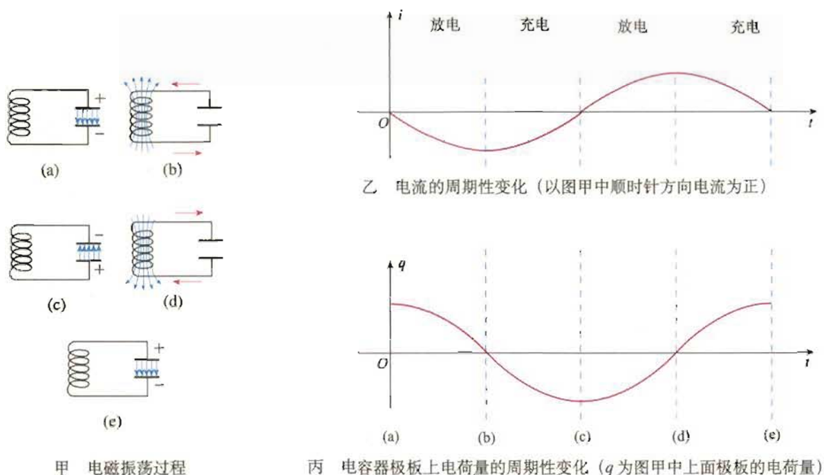
图 14.2-2 LC 振荡电路及其电流、电荷的变化
