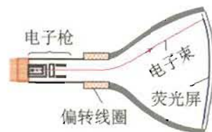
图 14.4-3 显像管
