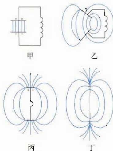
图 14.3-1 由闭合电路变成开放电路
