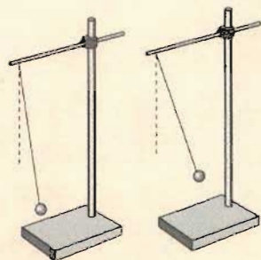
图 11.4-4 单摆振动的周期与什么因素有关?
