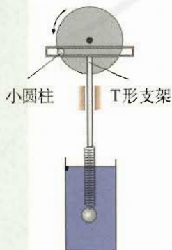
图 11.5-7 小球做受迫振动
