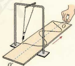
图 11.4-2 画出振动图象
