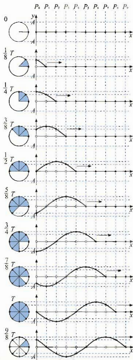
图 12.1-3 横波的形成
