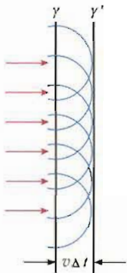
图 12.6-3 用惠更斯原理解释平面波的传播
