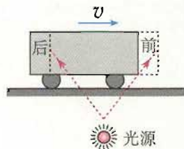
图15.2-6 车上人认为闪光先到前壁还是后壁?
