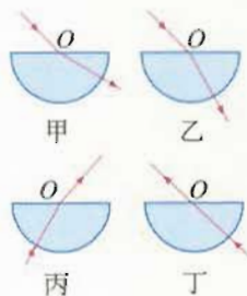
图 13.1-5 哪些情况可能发生?
