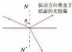
图 13.6-4 反射引起自然光的偏振
