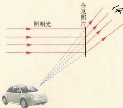
图 13.8-4 观察全息照片
