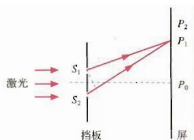
图 13.3-3 距离中心 P_0 点越远的点, 两条狭缝射来的光的路程差越大。
