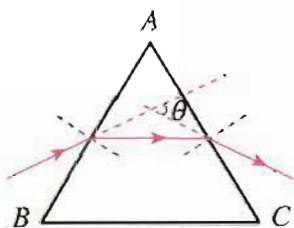
乙 光线通过棱镜的光路
