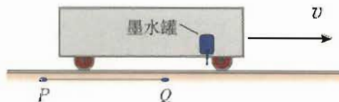
图 15.2-4 车上与车下的观察者认为两次滴水的的时间间隔不一样
