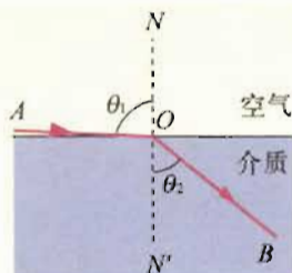
图13.2-2 首先计算光线掠射进入介质时的折射角
