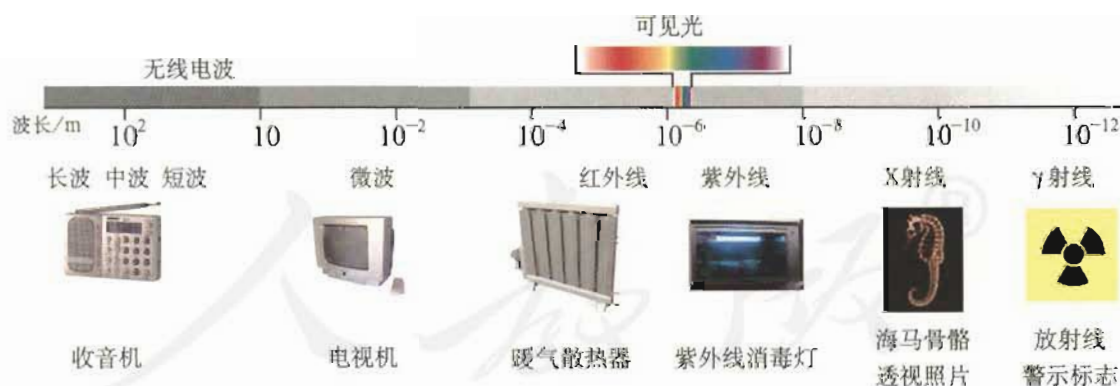
图 14.5-1 电磁波谱
