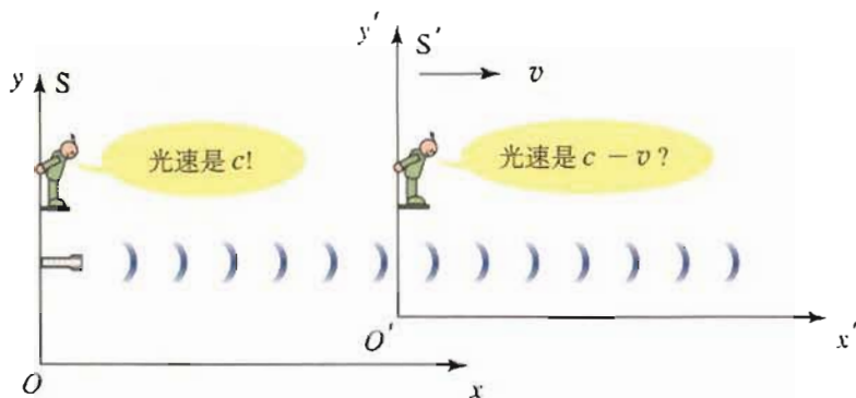
图 15.1-1 难道光的速度在两个参考系中不一样？
