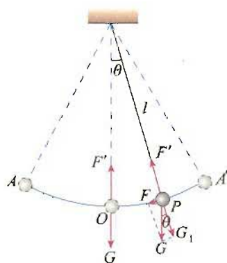
图 11.4-3 单摆的回复力
