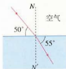
图 13.1-6 求介质的折射率
