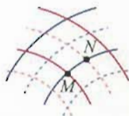
图12.4-7 两列频率相同的横波相遇
