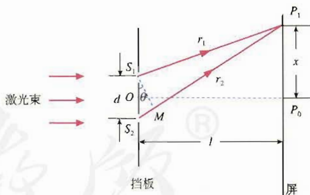
图 13.4-1 导出相邻亮条纹距离的表达式
