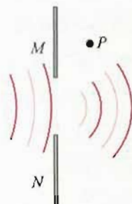
图12.4-6 水波衍射实验的俯视图
