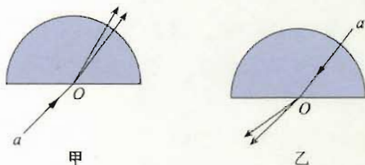
图 13.7-11 白光经过半圆玻璃砖后发生色散
