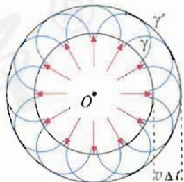
图12.6-2 用惠更斯原理解释球面波的传播
