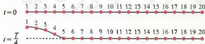
图 12.1-7 绳波的形成
