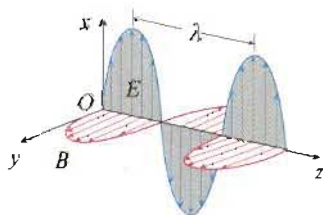
图 14.1-3 沿 z 轴传播的电磁波。与 z 轴垂直的箭头表示此时刻轴上各点的电场方向和磁场方向。
