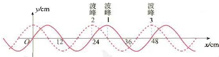
图 12.3-2 一列正弦波的波形曲线
