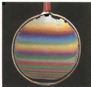
图 13.7-4 肥皂膜的干涉现象
