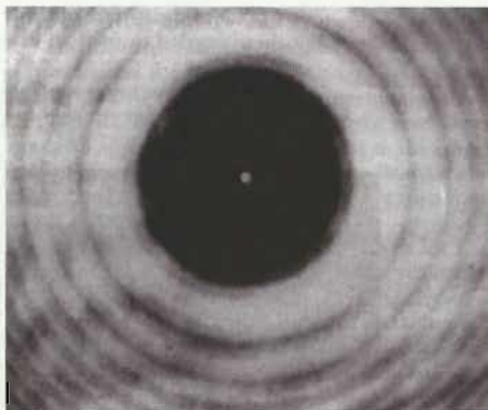
图 13.5-5 泊松亮斑
