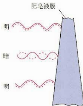
图13.7-3 薄膜前后两个面的反射光发生了干涉
