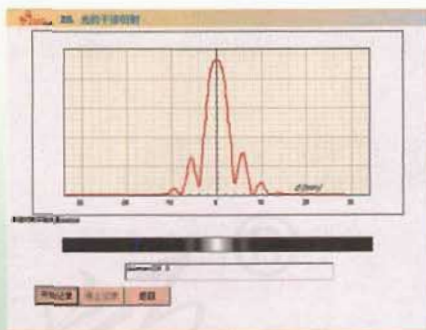
图13.5-4 单缝衍射图样和光强分布图象
