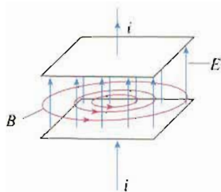
图 14.1-2 变化的电场产生磁场
