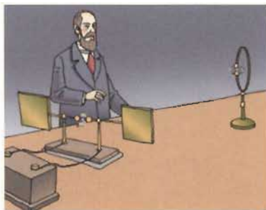
图 14.1-4 令人兴奋的电火花
