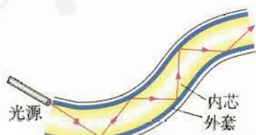
图 13.2-7 光导纤维
