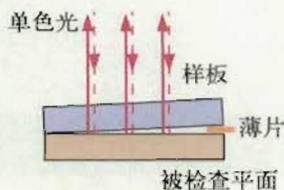
图 13.7-6 从样板的标准平面和被检查的平面反射的两列光发生干涉
