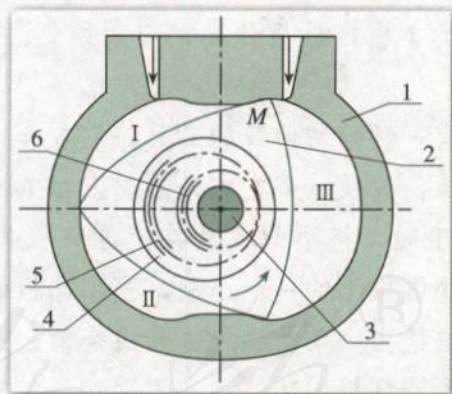
(旋转活塞发动机)
