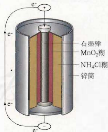
图 2-11 干电池构造示意图
