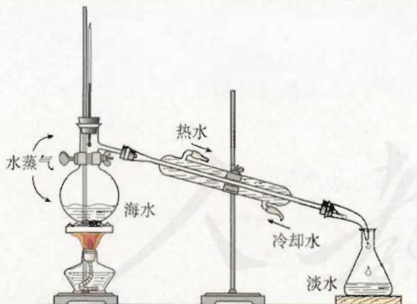
图 4-3 海水蒸馏原理示意图
