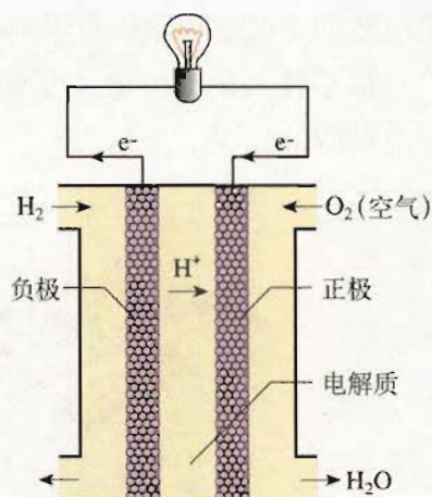
图 2-15 氢氧燃料电池构造示意图
