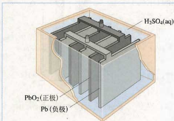
图 2-12 铅蓄电池构造示意图
