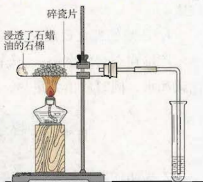
图 3-7 石蜡油分解实验
