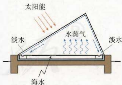
图 4-4 太阳能蒸发原理示意图
