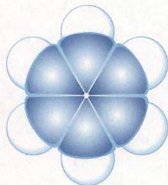
图 3-11 苯分子模型
