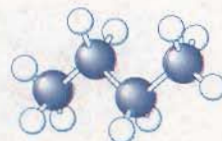
正丁烷
